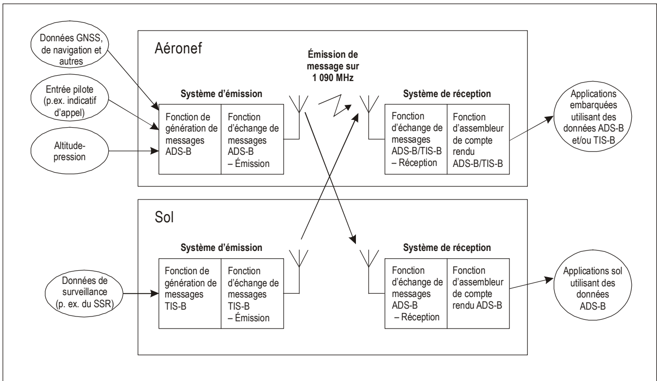
Figure 5-1. Modèle fonctionnel de système ADS-B/TIS-B
