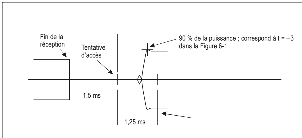
Figure 6-3. Temps de retournement réception-émission
