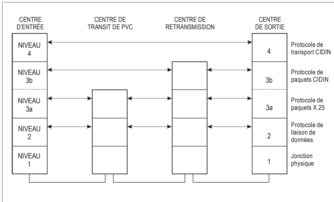
Figure 8-1. Niveaux de protocole CIDIN
